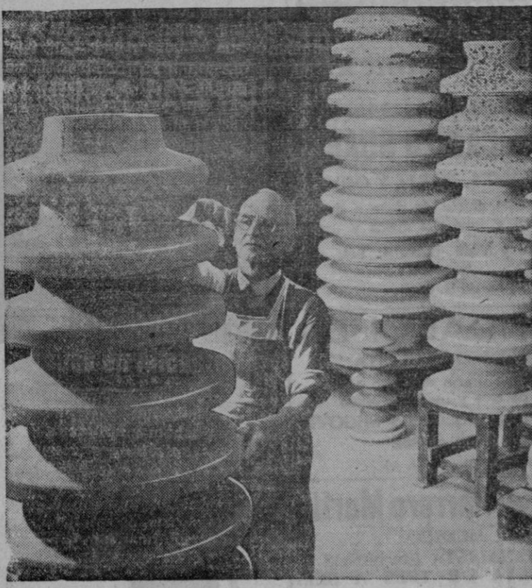
Sala de montaje de una fábrica de construcción de los mayores aisladores eléctricos de porcelana que se fabrican en Inglaterra. Parte de su producción se destina a los mercados de Ultramar
