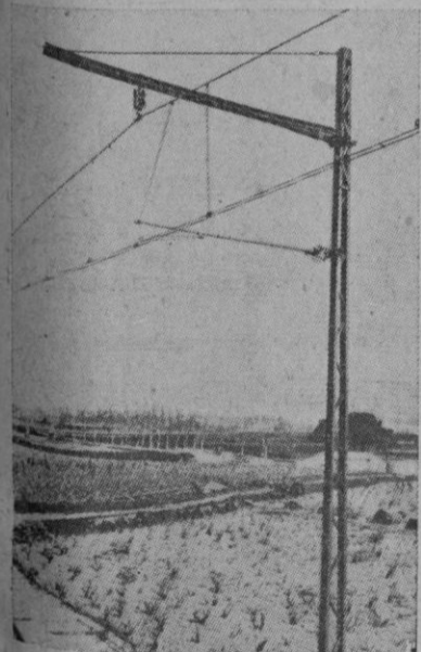
Castillete de hierro utilizado en la electrificación de la línea. El tipo de suspensión de esta línea es de catenaria simple, con doble hilo de contacto de cobre, colgado, por intermedio de péndolas, de un cable sustentador
