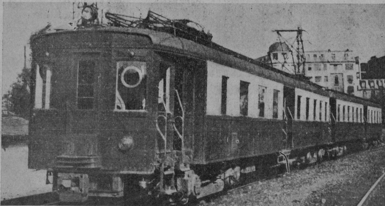
Una de las 30 «unidades de tren» construidas para la misma línea. Tiene una capacidad de 171 asientos y va provista de calefacción eléctrica y furgón de equipajes. La potencia de cada coche automotor es de 920 C. V. Con él pueden formarse trenes hasta de cuatro «unidades», o sean ocho coches
