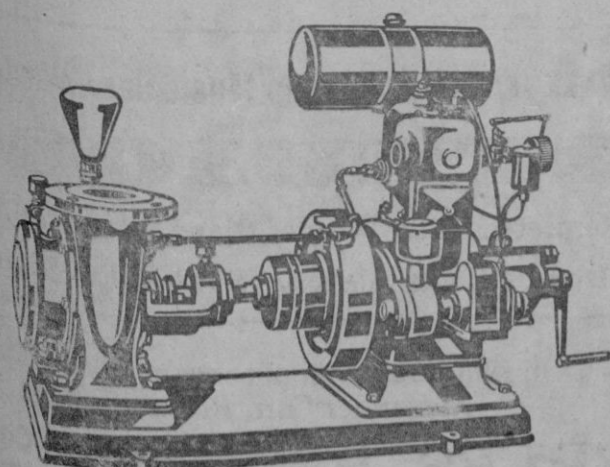
MOTO - BOMBA
