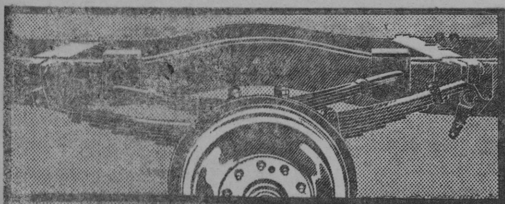
Las ballestas auxiliares traseras aseguran una mejor suspensión de la carga y una mayor estabilidad del camión.
