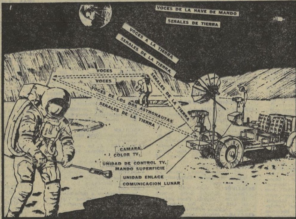
En el dibujo, esquema del sistema de transmisiones utilizado por los astronautas entre sí, y con la Tierra y módulo de mando
