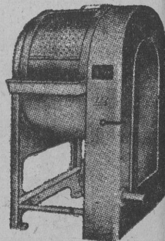
LAVADORA PARA ROPA (modelo industrial) Se fabrican de 6 a 100 kgs. Reversibilidad automática. Gran rendimiento
