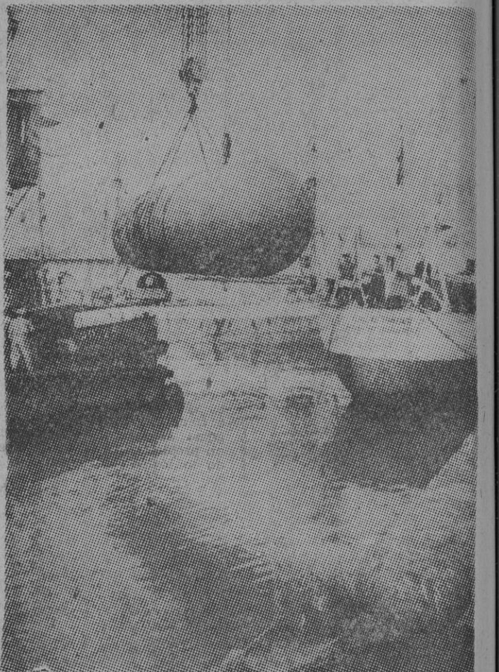
PALMA DE MALLORCA: Uno de los grandes tanques para almacenamiento de gas butano-propano, construido por una factoría de Tarragona y con destino a la planta de embotellado que se está instalando en Alcudia (Mallorca), es descargado en el puerto de Palma.
