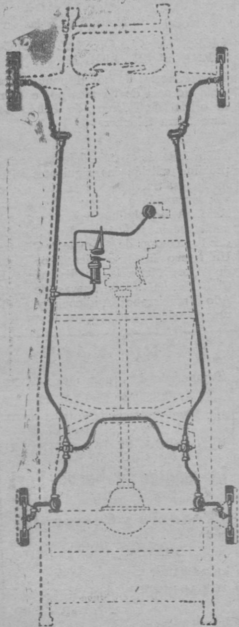
Diseño de un chasis Paige Jewett de frenos hidráulicos 4 ruedas, ataque directo sin conexiones ni mandos complicados en absoluto de puntos que deban engrasarse.
