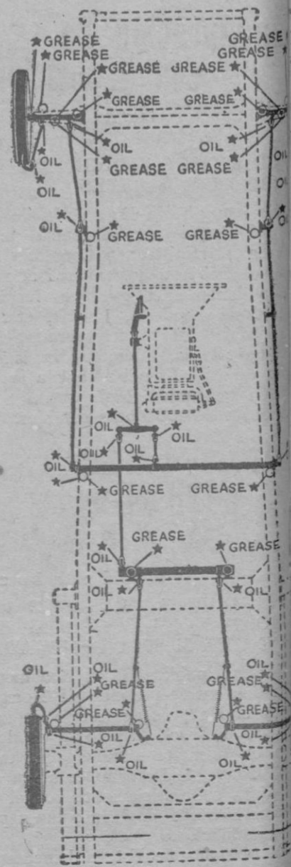
Diseño de un chasis con frenos hidráulicos 4 ruedas de men los mecánicos y los que deben engrasarse.
