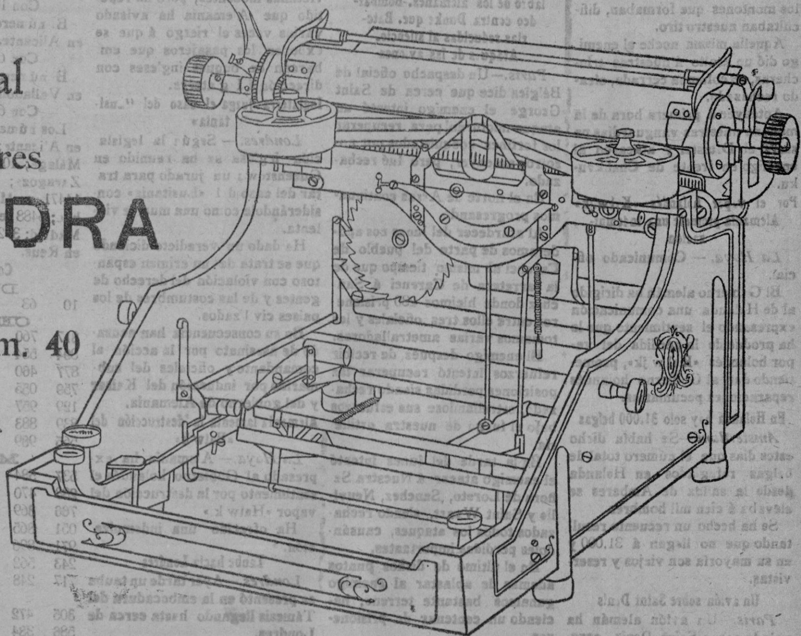
La máquina sin la cesta de tipo. La única máquina con la cesta de tipo movable.
