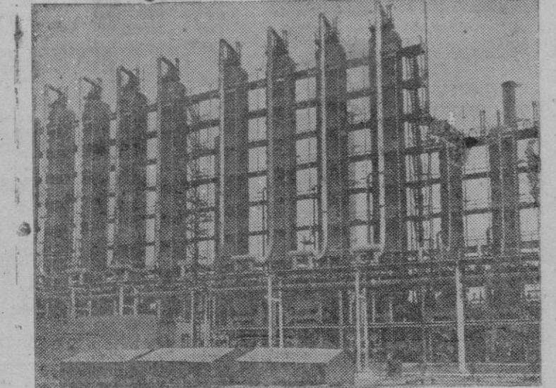
UNA FABRICA DE TOLUENO NORTeamericana. — En esta red de torres, tubos y depósitos que se eleva a una altura de 10 metros sobre el suelo, en el Sudeste de los EE. UU., el petróleo se convierte en tolueno, ingrediente fundamental del TNT, uno de los explosivos más potentes.
