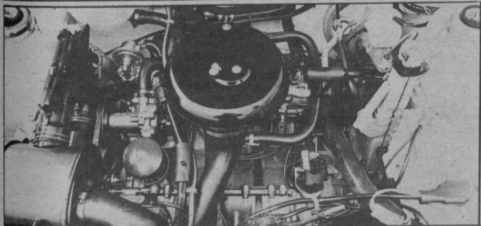
En el vano motor se puede trabajar cómodamente, una vez quitada la rueda de repuesto que va encima del filtro del aire. El motor va muy inclinado, casi plano respecto a la horizontal.
