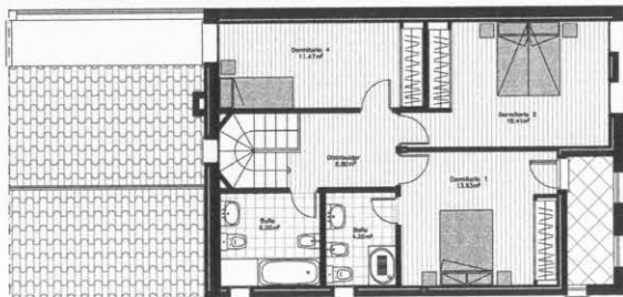
PLANTA ALTA
