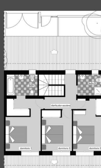
Planta primera
