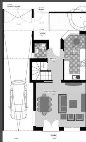
Planta baja
