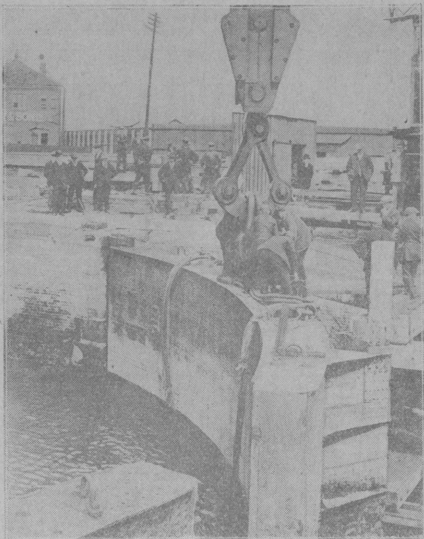
Colocación de un enorme bloque de 140 toneladas en dos horas en el grandioso muelle Reina Victoria, cuyas obras están siendo realizadas con grandísima rapidez dados los grandes medios de que disponen.
