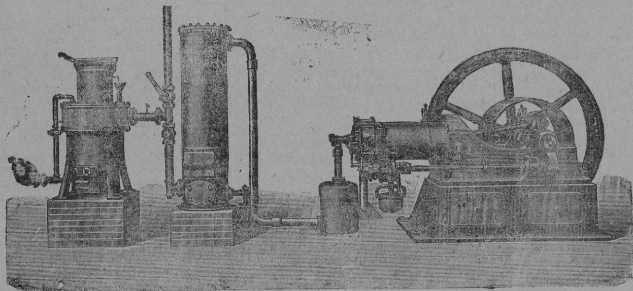
Motores de gas combinados con fábrica de GAS POBRE del nuevo sistema por aspiración. Más de 100 instalaciones funcionando en España (en Mallorca 4). La fuerza motriz más económica de la actualidad.
