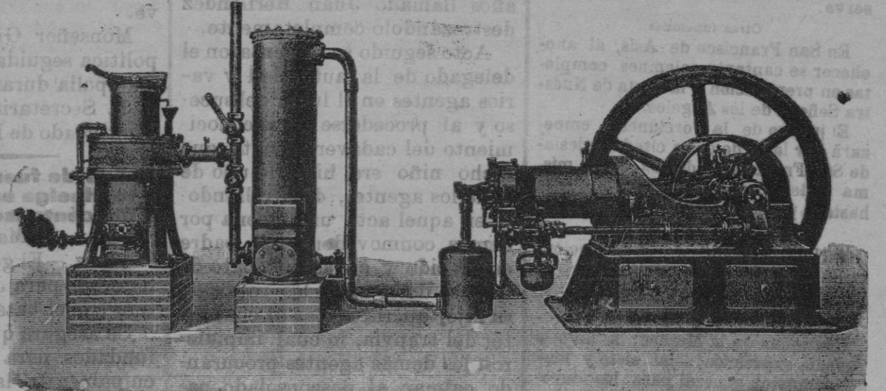
Motors de gas combinados con fábrica de GAS POBRE del nuevo sistema por aspiración. Mas de 100 instalaciones funcionando en España (en Mallorca 4). La fuerza motriz más económica de la actualidad.
