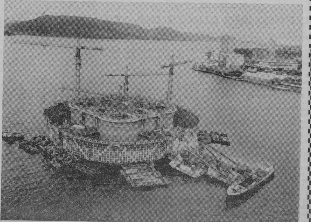
PARA ALMACENAR EL PETROLEO QUE SERA EXTRAIDO DEL YACIMIENTO DEL MAR DEL NORTE SE ESTA CONSTRUYENDO ESTE INCREIBLE ALMACEN MARITIMO PARA SER COLOCADO SOBRE "EL TERRENO" PETROLIFERO. TENDRA UNA CAPACIDAD PARA UN MILLON DE BARRILES EN PLENO MAR
