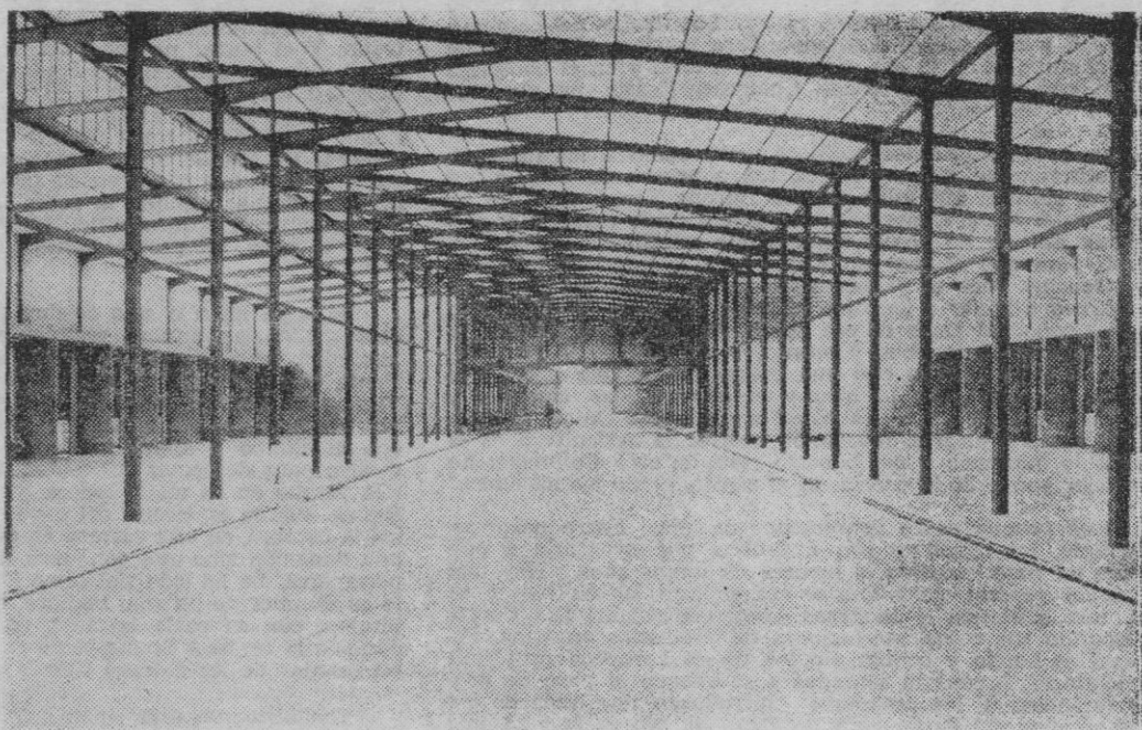
INTERIOR DE UNA DE LAS NAVES DEL PABELLON DE FRUTAS Y VERDURAS EN EL QUE SE APRECIA EL AVANZADO ESTADO DE LAS OBRAS, PENDIENTES UNICAMENTE DE LOS ÚLTIMOS DETALLES. - (Foto JUANET)
