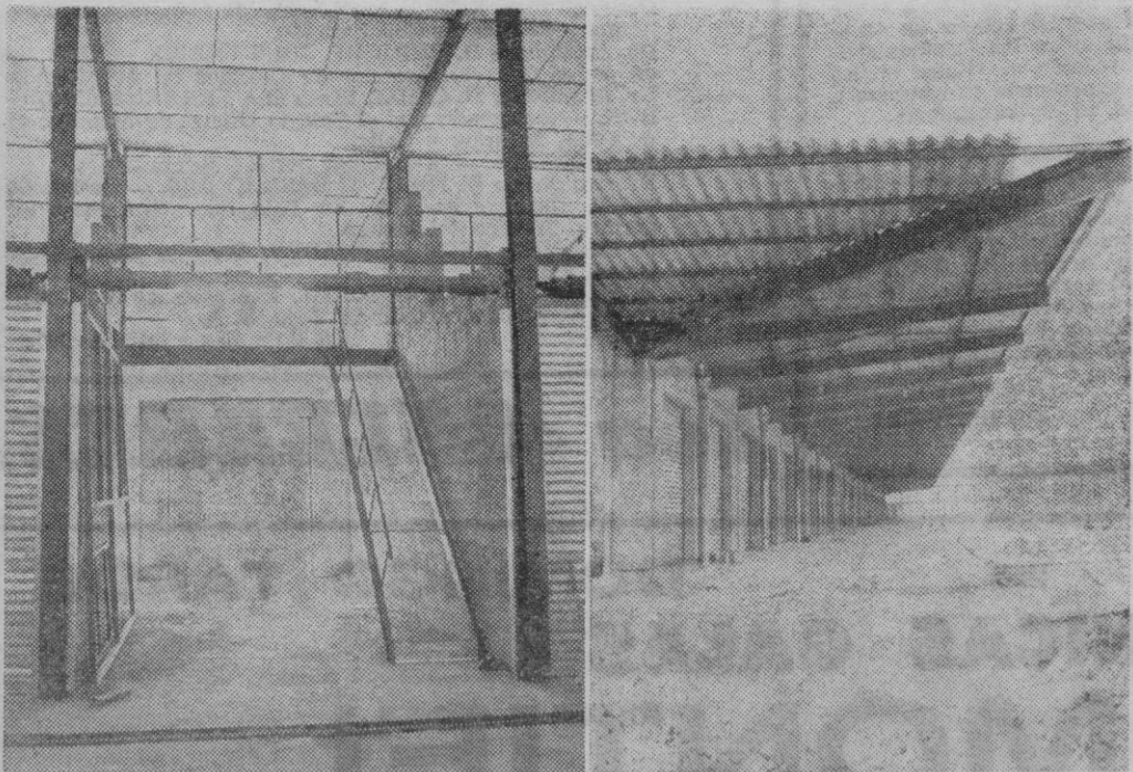
INTERIOR DE UNO DE LOS PUESTOS DE ASENTAMIENTO DE MAYORISTAS, CON INSTALACION FRIGORIFICA COMPLEMENTARIA Y VISTA LATERAL DE UNO DE LOS ANDENES DE DESCARGA DE LOS PABELLONES ACTUALMENTE EN CONSTRUCCION. - (Foto JUANET)
