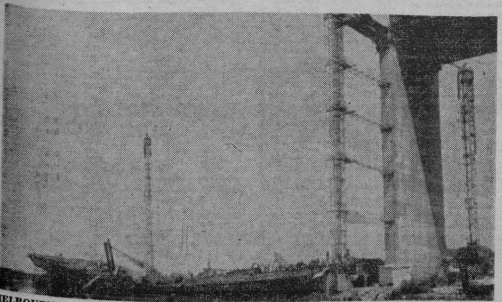
MELBOURNE. -- Hierros retorcidos y otros destrozos, tras derrumbarse parcialmente el puente en construcción de la autopista de Westgate, sobre el río Yarra. Dos horas después del derrumbamiento fueron hallados diecinueve cadáveres entre el barro y los escombros. (Telefoto UPI-CIFRA)
