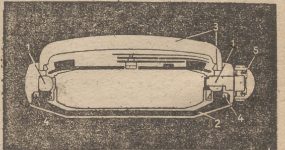
1 - JUNTA ELASTICA 3 - CRISTAL ARMADO 2 - FONDO DE ACERO 4 y 5 - JUNTAS IMPERMEABLES ROSCADO
