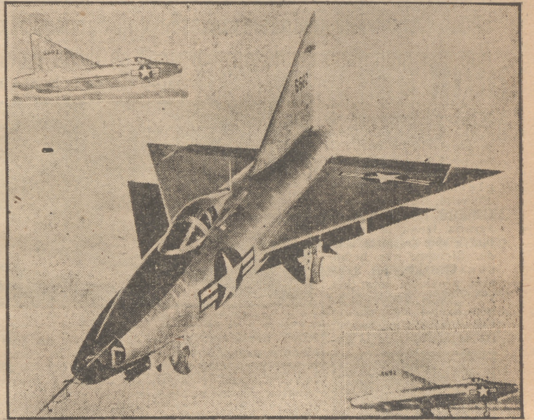
Las fuerzas aéreas norteamericanas poseen el nuevo modelo F-100, con alas triangulares, impulsado a chorro. El aparato ha sido probado con éxito en la base aérea de Muroc (California), y fue construido para experimentar el sistema superioridad en este tipo de aparato sobre los ya conocidos. Los técnicos dicen que obtiene mayor velocidad y menor resistencia al aire y que puede alcanzar grandes velocidades supersonicas.
