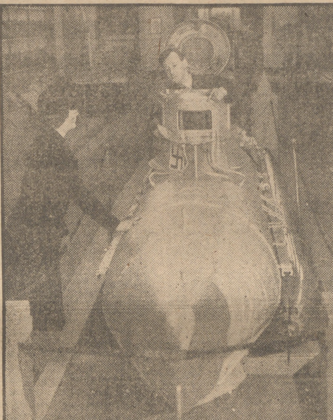
En el Museo Imperial de la Guerra, en Hamburgo, figura este submarino monoplaza empleado por los alemanes. Llevaba dos torpedos de 21 pulgadas. Su radio de acción era de 75 millas en superficie y 12 sumergido. Podía sumergirse a 150 pies. Sus dimensiones son: 29 pies y cuatro pulgadas de largo y tres pies seis pulgadas de ancho, sin los torpedos, que van a los costados. (Foto A. P.)
