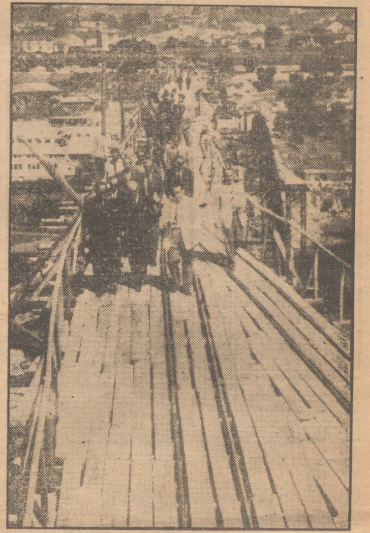
El señor Fernández Ladreda recorre el viaducto que se construye sobre el Miño para el ferrocarril Zamora-La Coruña. (Foto Cifra.)
