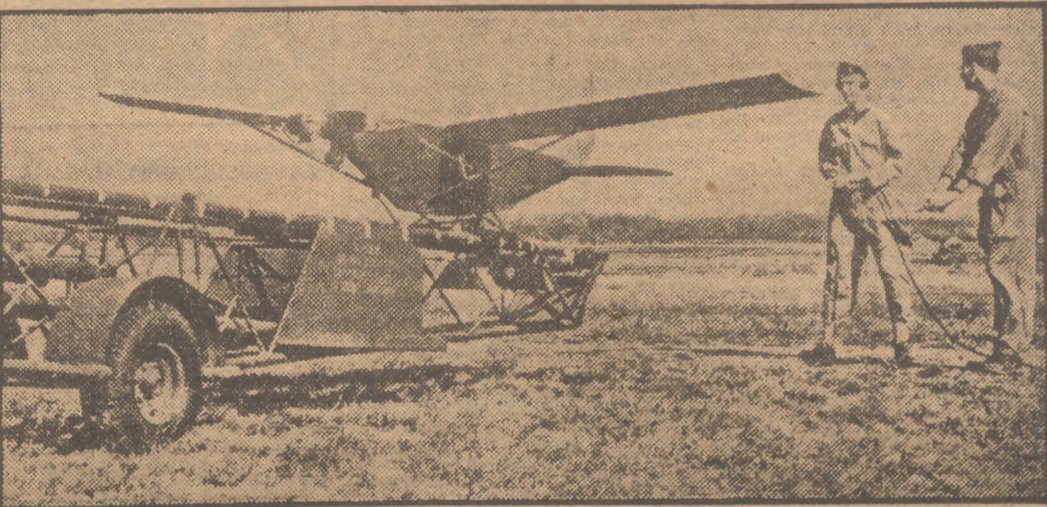
Un avión de bombardeo sin piloto. Momento de ser lanzado en la catapulta por onciales del Ejército americano, el avión sin piloto, dirigido por radio, que después de descargarse una bomba de 20.000 libras regresa a su base, descendiendo en para caídas.
