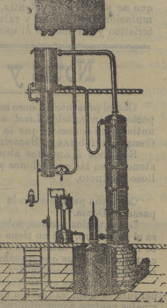
Aparato de rectificación.
