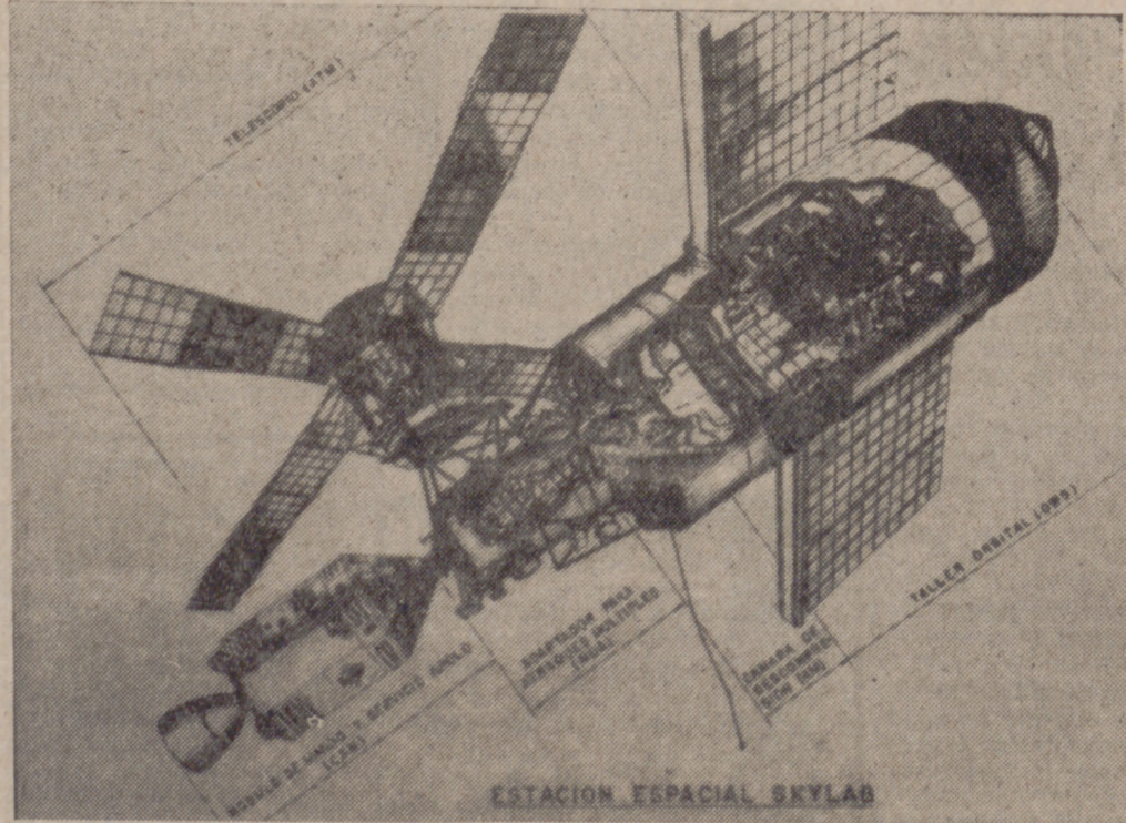
La Estación Espacial Skylab tiene por finalidad aumentar los conocimientos sobre vuelos tripulados en órbita terrestre, y llevar a cabo investigaciones de orden científico, técnico y medio.—(Foto PYRESA.)
