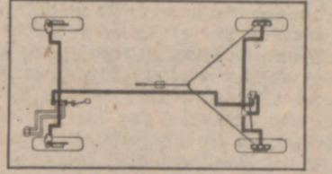
Circuito de frenos dobles e independientes. Corrector de frenada sobre las ruedas posteriores.
