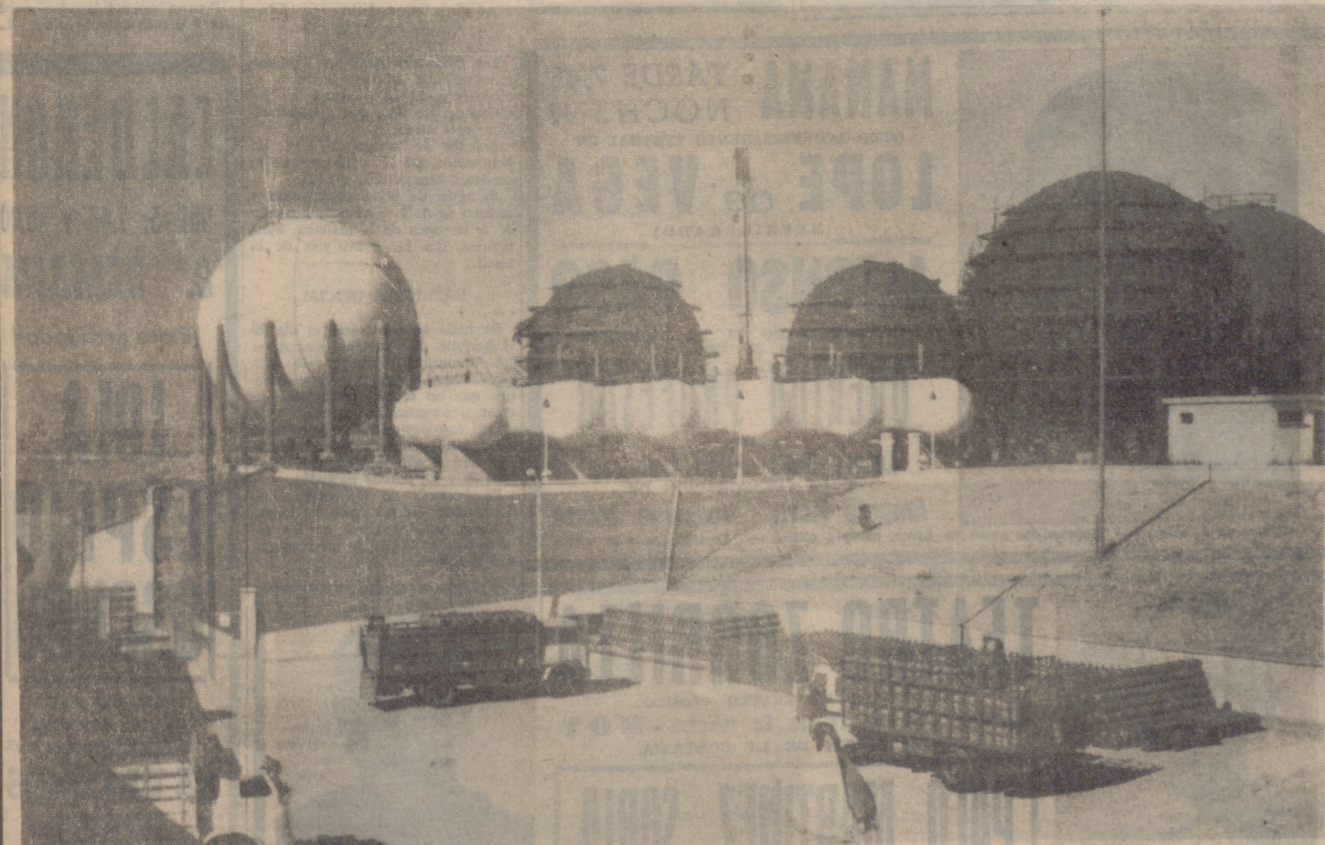
Planta de embotellado de Venta de Baños, con esferas de 2.000 metros cúbicos y tanques de 213 metros cúbicos.
