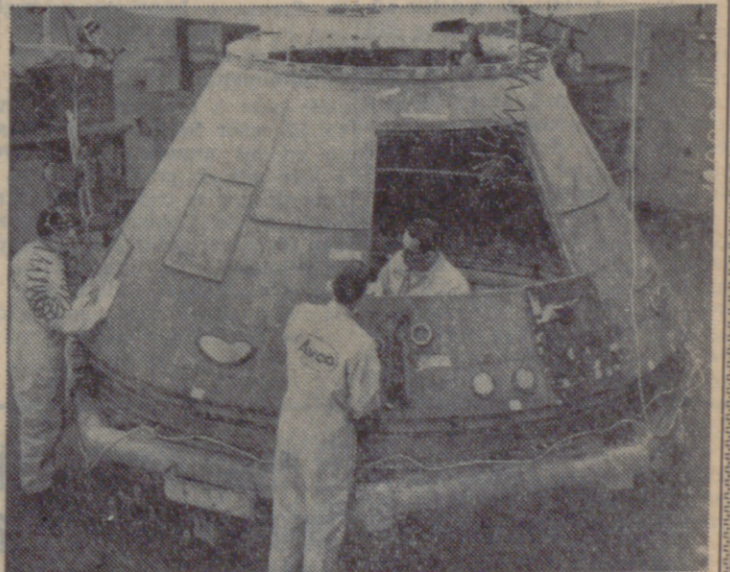
Tres expertos de la fábrica AVCO, de Lowell (Massachusetts) terminan de armar el blindaje térmico para la astronave "Apolo". El blindaje se compone de 350.000 celdas a manera de panel, llenas de un material aislante, y protegerá a los tres astronautas de la tripulación del efecto de las temperaturas sumamente altas generadas por la fricción atmosférica durante el trayecto de regreso de la nave a la Tierra después de su vuelo de exploración lunar.
