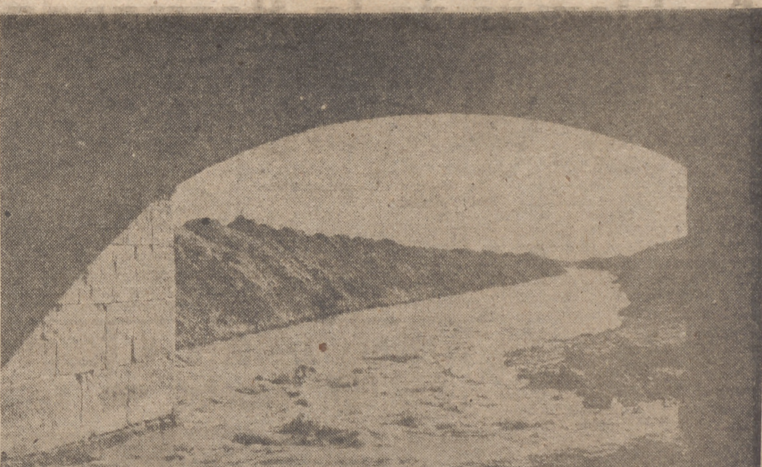
Puente de Villafuerte, mirando hacia aguas abajo. Se observa en el centro de la foto una fuerte velocidad, como si la rasante cambiara precisamente en la obra de fábrica. Por lo visto, un problema viejo de cuando los pueblos, por su cuenta y sin consultas, hacían las mondas o limpiezas por su cuenta.
