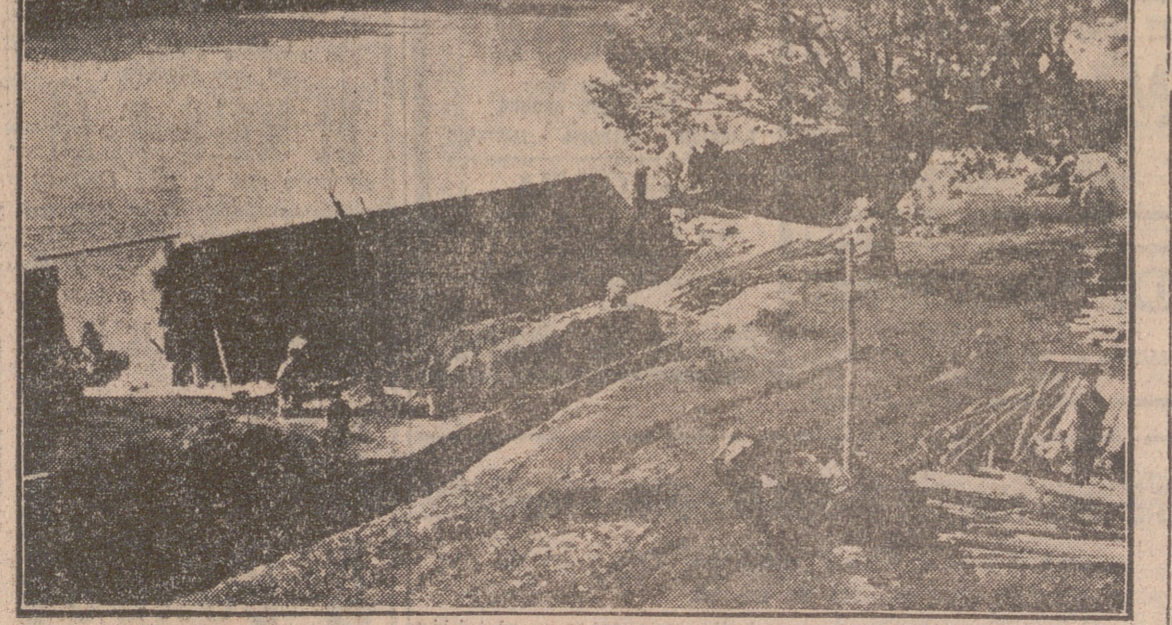
Inmediatamente de adjudicarse por el Ayuntamiento las obras de construcción de los puentes sobre el Pi-suegra, las obras han dado comienzo. La rapidez ha causado tanta sorpresa como satisfacción, y en la "foto" de Carvajal vemos los primeros trabajos de construcción del puente que se elevará en la parte de "El Cubo". El muro de contención del río ha sido abierto; los árboles, talados; las edificaciones, destruidas, y la zanja de cimientos, comenzada. Así da gusto. Hay quienes sueñan ya en darse un paseito por el nuevo puente el próximo verano. ¡Que se a realidad su deseo!
