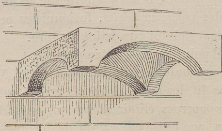
Fig. 1. — Porche de l'église de Moissac.
