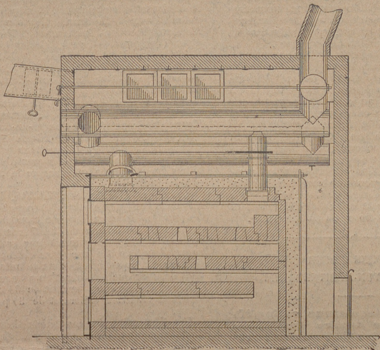
Fig. 1 - Coupe longitudinale
