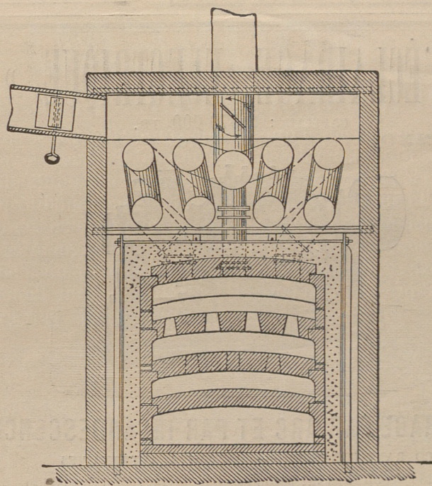
Fig. 2 - Coupe transversale
