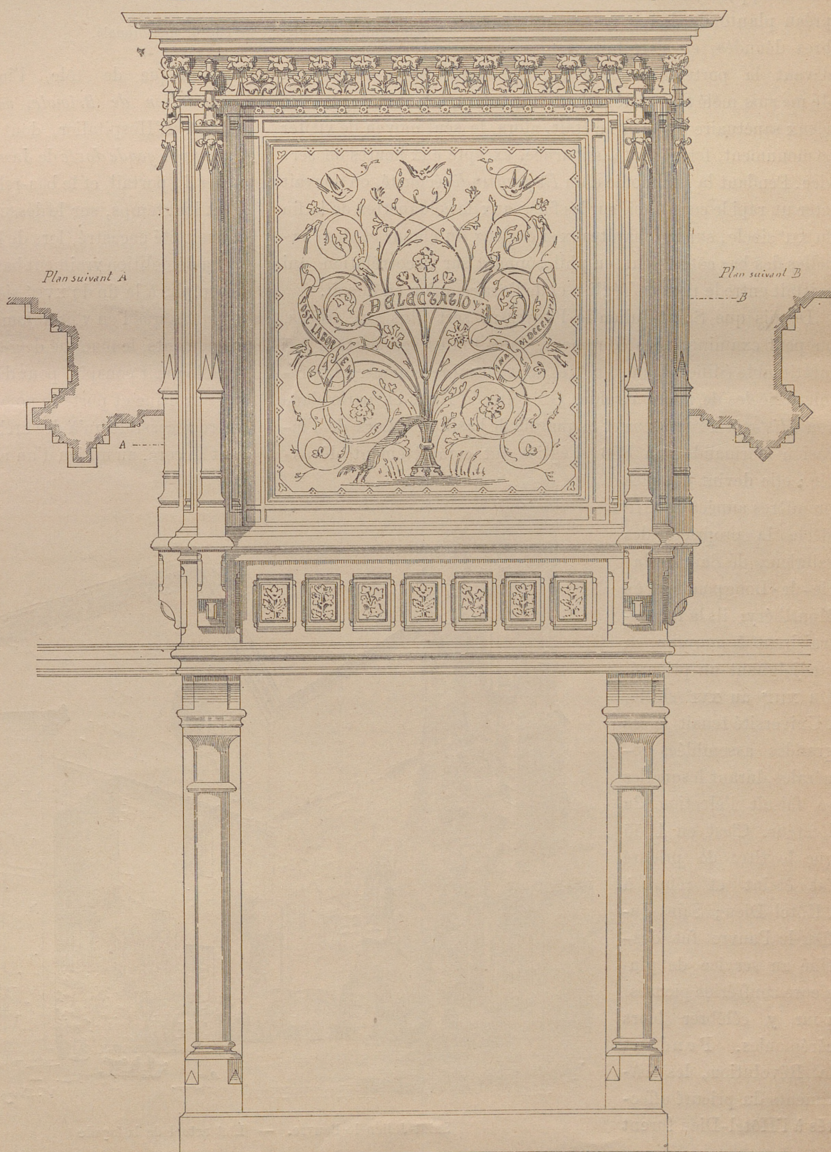
VILLA A SAINT-JAMES. — Cheminée de la salle à manger.
