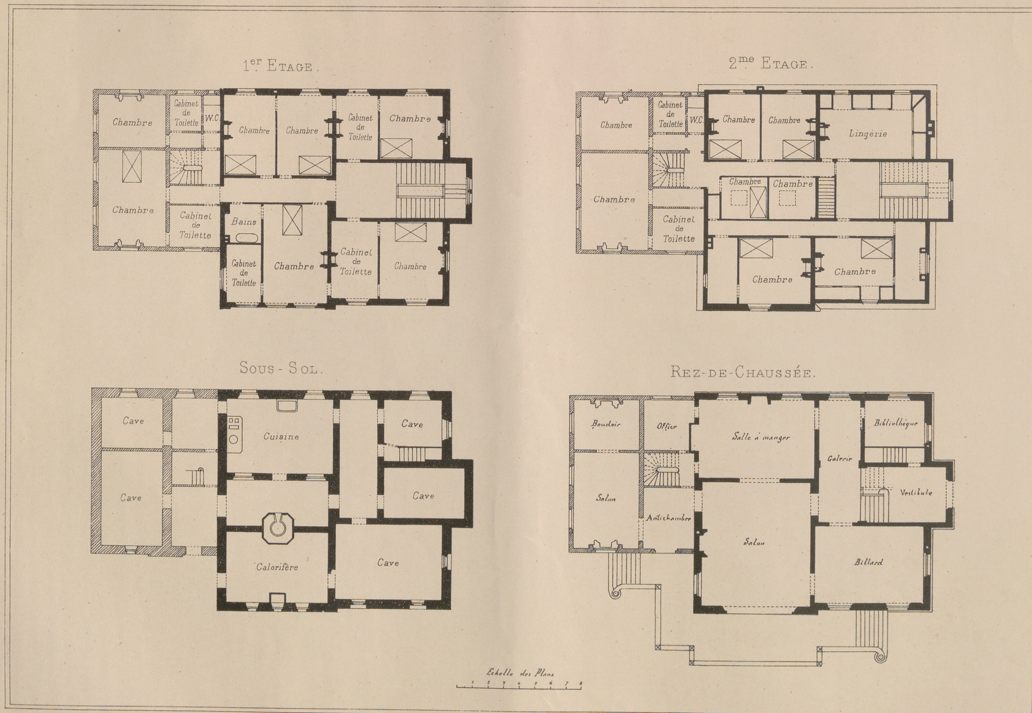
VILLA à S t JAMES (Seine). ARCH: M. AUBRY.
