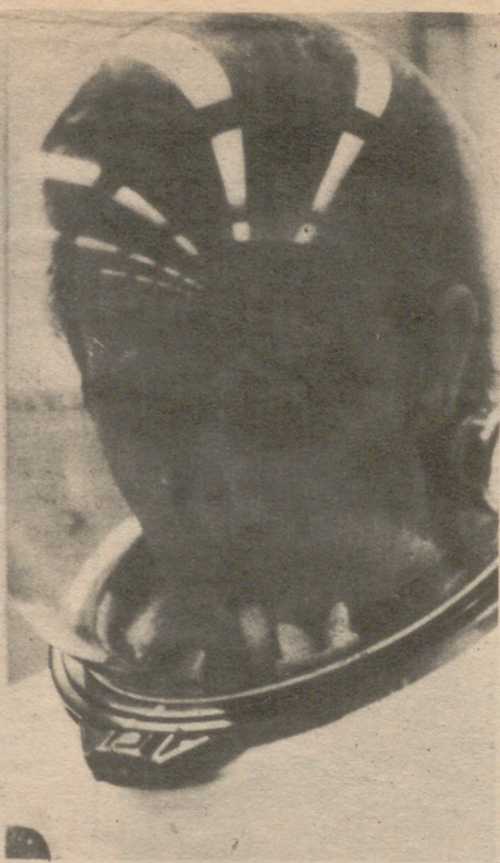
HOUSTON. Primer plano del prototipo del saco de agua del Apolo XIII (izq.) que será usado por los astronautas durante la misión lunar del Apolo. Ha sido probado por Walter D. Salyer, Jr., recientemente. Irá montado en la parte centro-derecha del casco y con un tubo servirá para que los astronautas tomen un trago de agua sin mover la cabeza.
