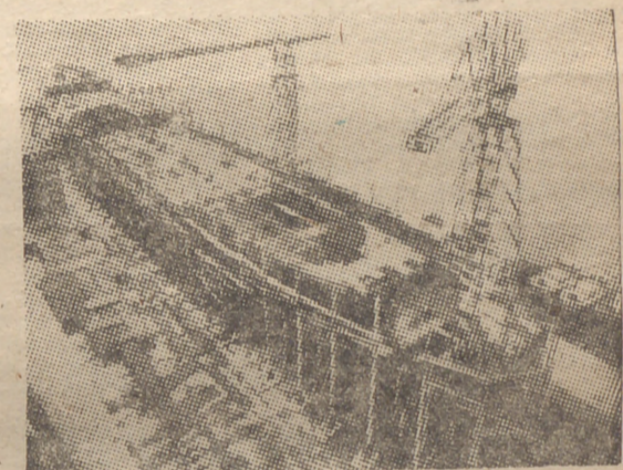
EL FERROL DEL CAUDILLO.—Petroleiro «Almirante F. Moreno», de 14.000 toneladas, en gradas, construido por la Empresa Nacional «Bazán»
