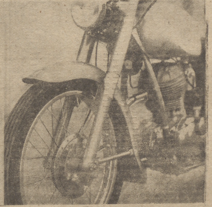
Indudablemente, la OSSA 175 c. c. es una de las máquinas mejor pensadas y llevadas a efecto en toda la producción motociclista mundial, como se aprecia en la factura de todos sus elementos.
