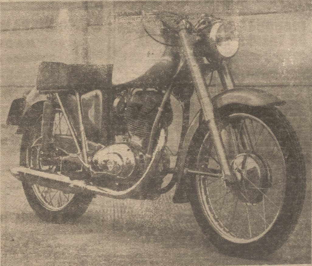
La actividad ciclista y motor de la OSSA 175 c. c. G. T. de cuatro tiempos, y la belleza de su trazado, se complementan con un atractivo y pulcro azul metalizado y cromados de perfecta ejecución.
