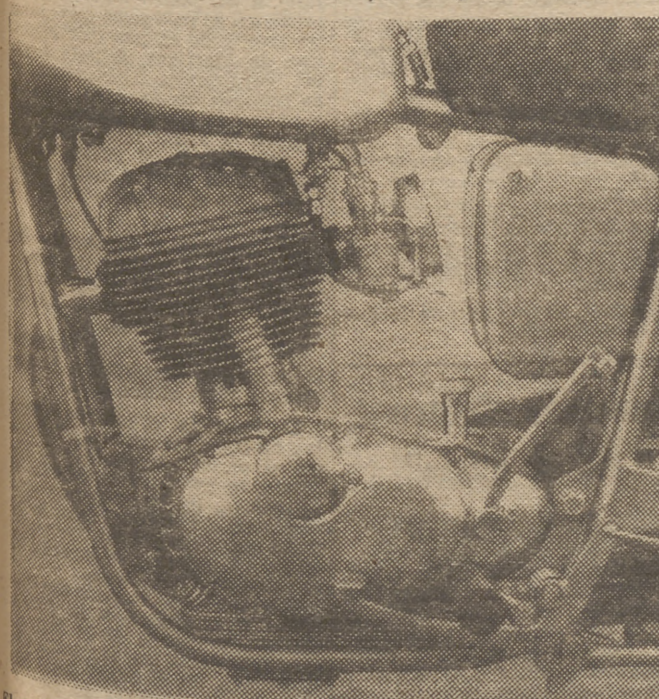
El cilindro, ligeramente inclinado para mejor refrigeración de la culata. La elegante concepción y cuidada realización del conjunto motor son signos clásicos en los productos OSSA.
