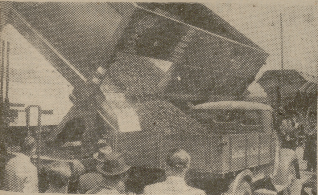
En la estación de Offenbach, los ferrocarriles alemanes han comenzado a utilizar este nuevo tipo de vagón de mercancías, de gran capacidad de carga y especialmente contruidos para el transporte de minerales. Los dispositivos de descarga automática permiten un ahorro de tiempo y mano de obra, gracias a la rapidez de la maniobra. (Foto Keystone-Nemes.)
