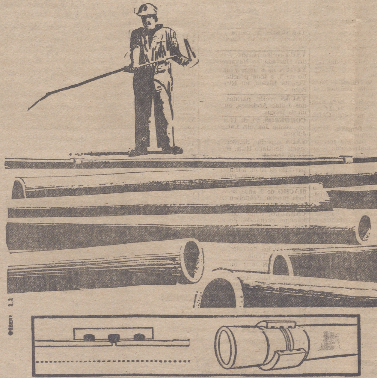
ESQUEMA DE COLOCACION DE LAS JUNTAS IBERIT. Disponemos también de toda la gama de piezas accesorias de fundición.
