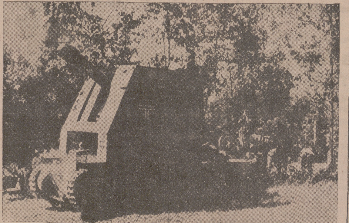
Cañón pesado alemán montado sobre el chasis de un tanque—dotado de gran movilidad—disparando desde el frente italiano.
