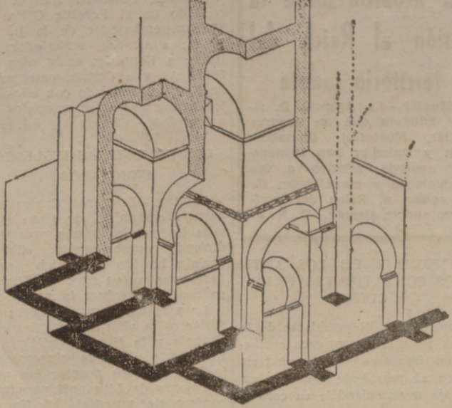
SANTA MARIA DE WAMBA.—Perspectiva isométrica del edificio
