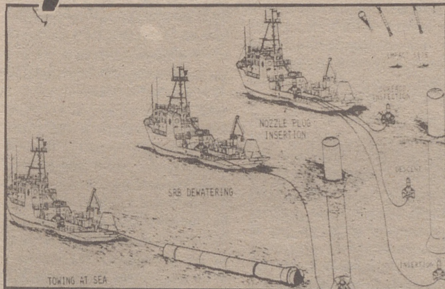
CENTRO ESPACIAL KENNEDY (Florida). — Gráfico facilitado por la NASA, en el que se explica las distintas fases para la recuperación del cohete impulsor de la nave espacial Columbia, reutilización se efectuará el viernes. (Telefoto Efe - AP)
