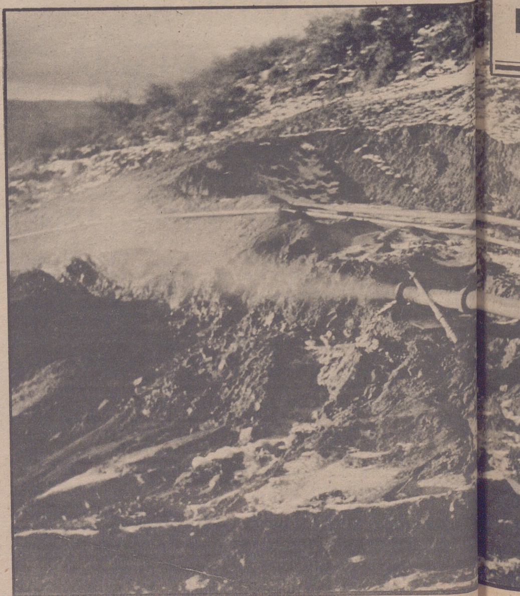
Tubería de pruebas. El gas aflora mezclado todavía con numerosas inmundicias
