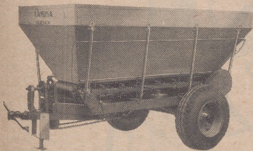
ABONADORA CENTRIFUGA Tipo remolque, de 2.250 kilos Homologada por el Ministerio de Agricultura
