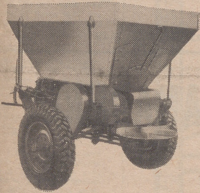
ABONADORA CENTRIFUGA Tipo remolque, de 1.000 kilos
