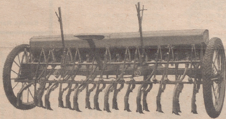
SEMBRADORA CUBRESEMILLAS DE CEREALES Modelo B-2 Tipos de 9, 12, 15, 18, 21 y 24 bocas
