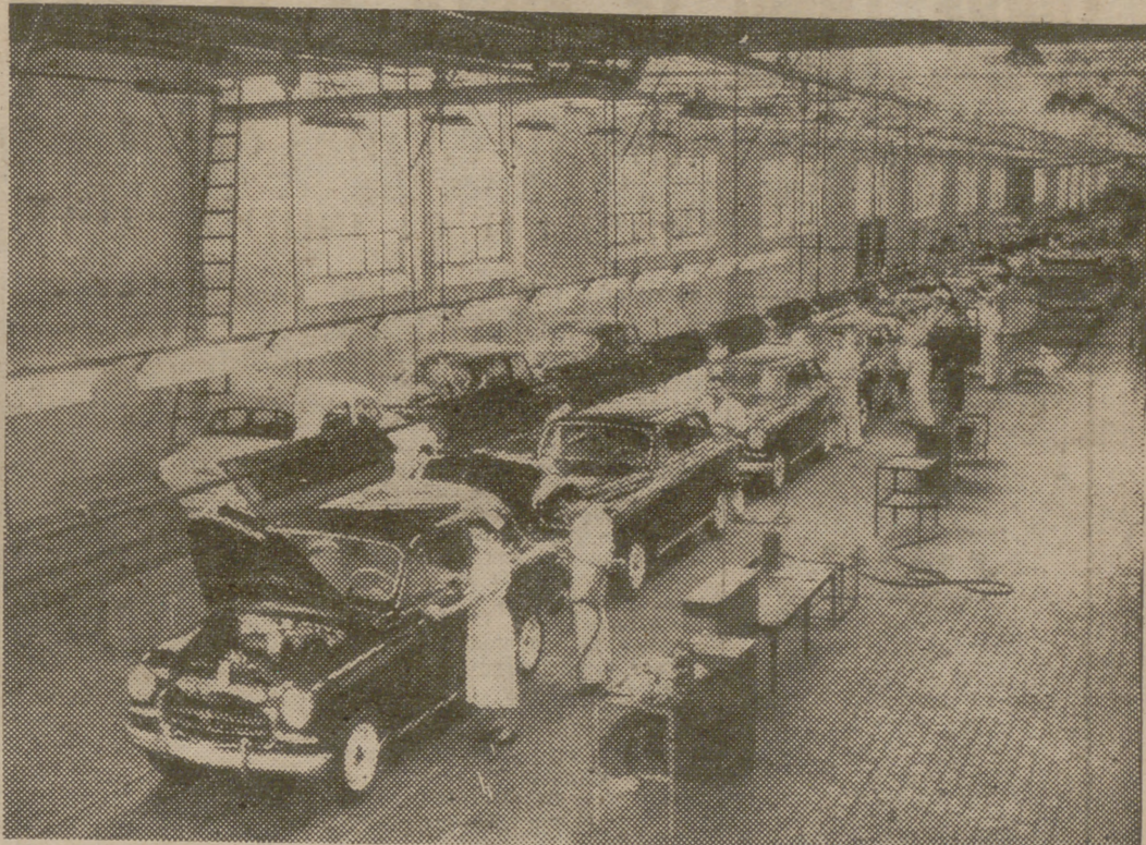
Vista parcial del taller de carrocerías. Cadena de acabado final
