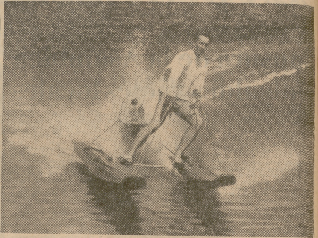
No sabemos si la innovación restará belleza al deporte del esquí acuático; sin embargo, no es poca cosa la ventaja que parece ofrecer el llamado "seasky", ideado en París para prescindir de la canoa de remolque. El aparato consiste en un par de flotadores accionados por un pequeño motor, que para automáticamente en caso de caída del piloto. El ingeniero inventor, M. Rouco, que aparece en la foto durante una de las pruebas del modelo, ha estado, al parecer, en todos los detalles. (Foto Cifra.)
