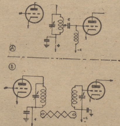
Figura 182.—Circuito transmisor
