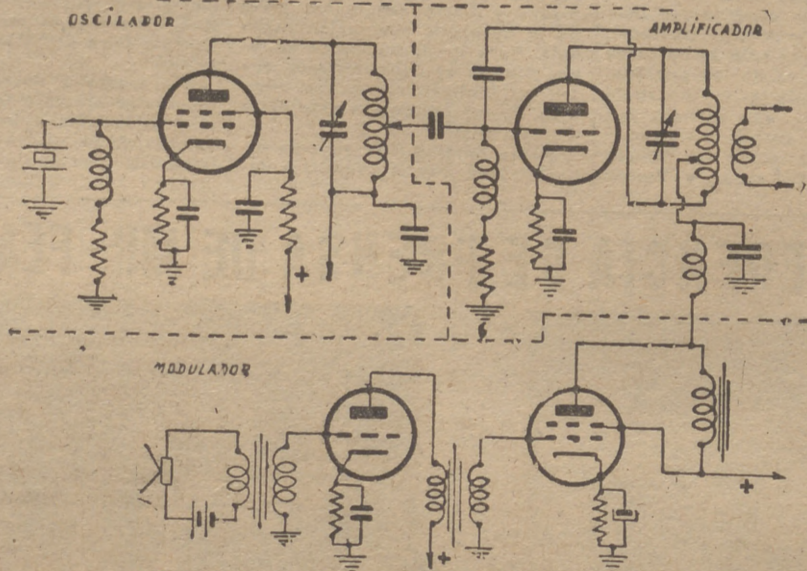
Figura 181.—Acoplamientos entre etapas
