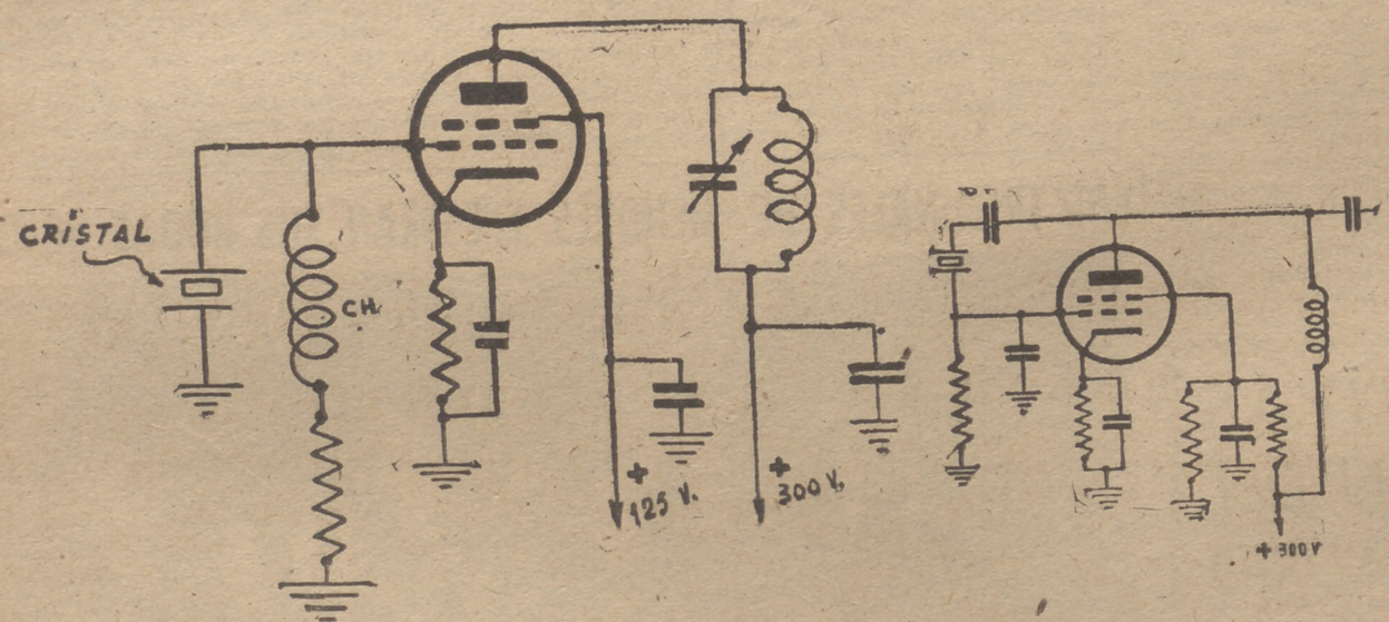
Figura 179.—Oscilador controlado a cristal
