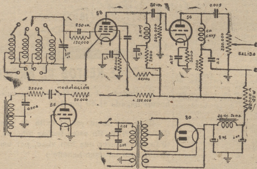
Fig. 144.—Esquema de un generador de señales.
